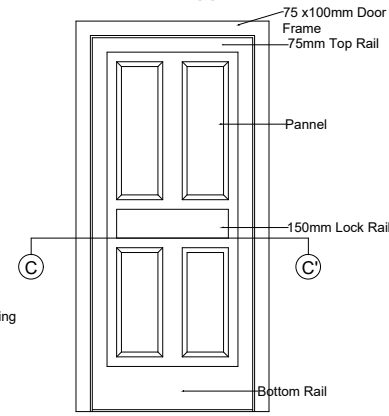
PANNELLED DOOR
