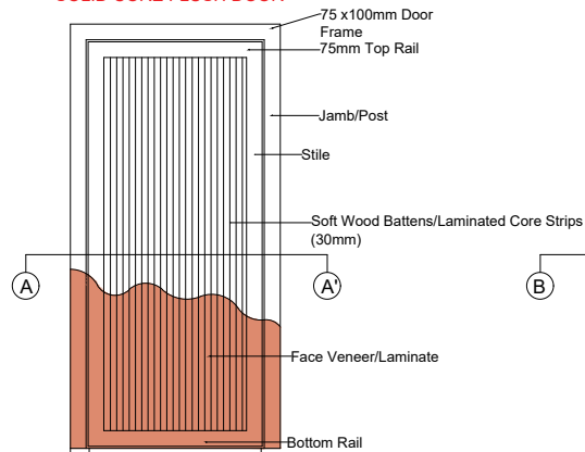
SOLID CORE FLUSH DOOR
