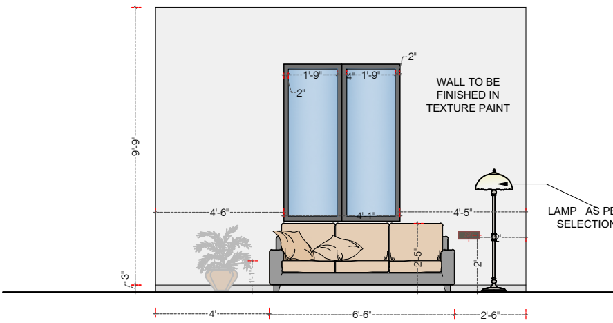
WALL B- ELEVATION
