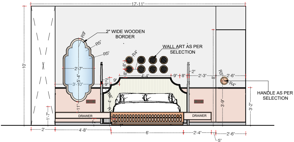
WALL A- ELEVATION
