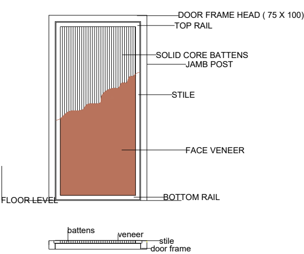
SOLID CORE FLUSH DOOR
