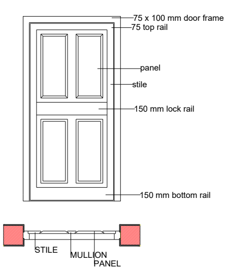
PANEL DOOR
